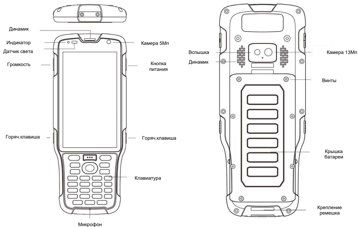
Рисунок 1.2 Внешний вид контроллера TC50
