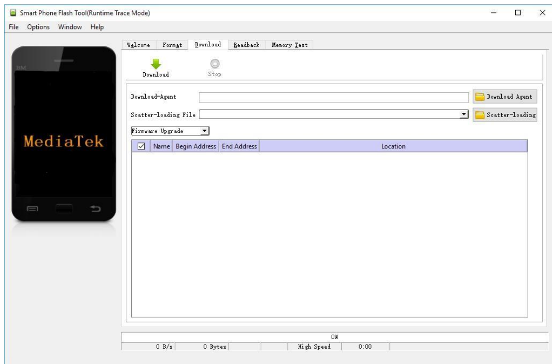
Рисунок 2.22 Интерфейс утилиты
