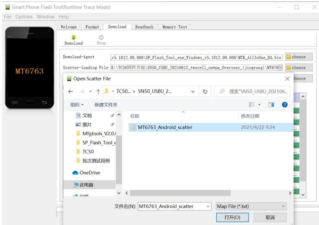
Рисунок 2.25 Загрузить Scatter-файл
