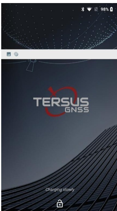
Рисунок 2.16 Слайд вверх
